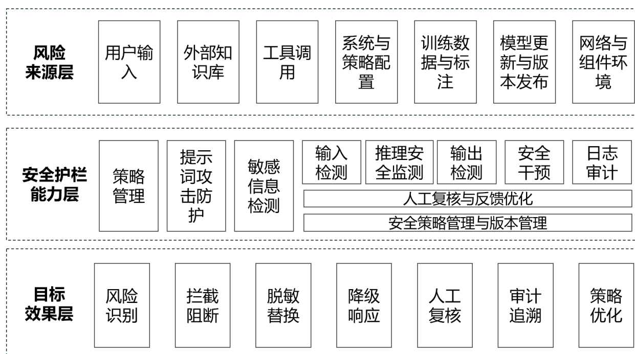
图 1 大模型安全护栏功能框架示意图
