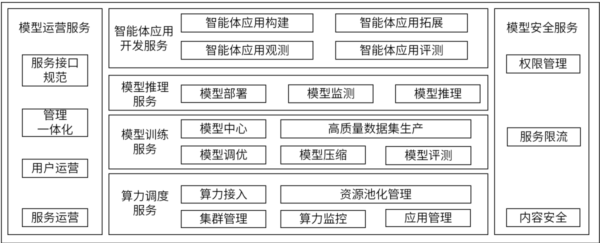
图 1 政务领域人工智能大模型统一服务平台成熟度模型框架
