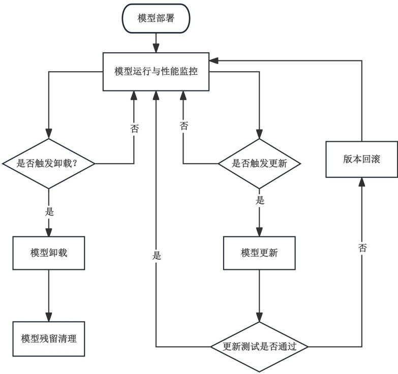
图 1 端侧大模型更新与运维总体流程逻辑示意图
